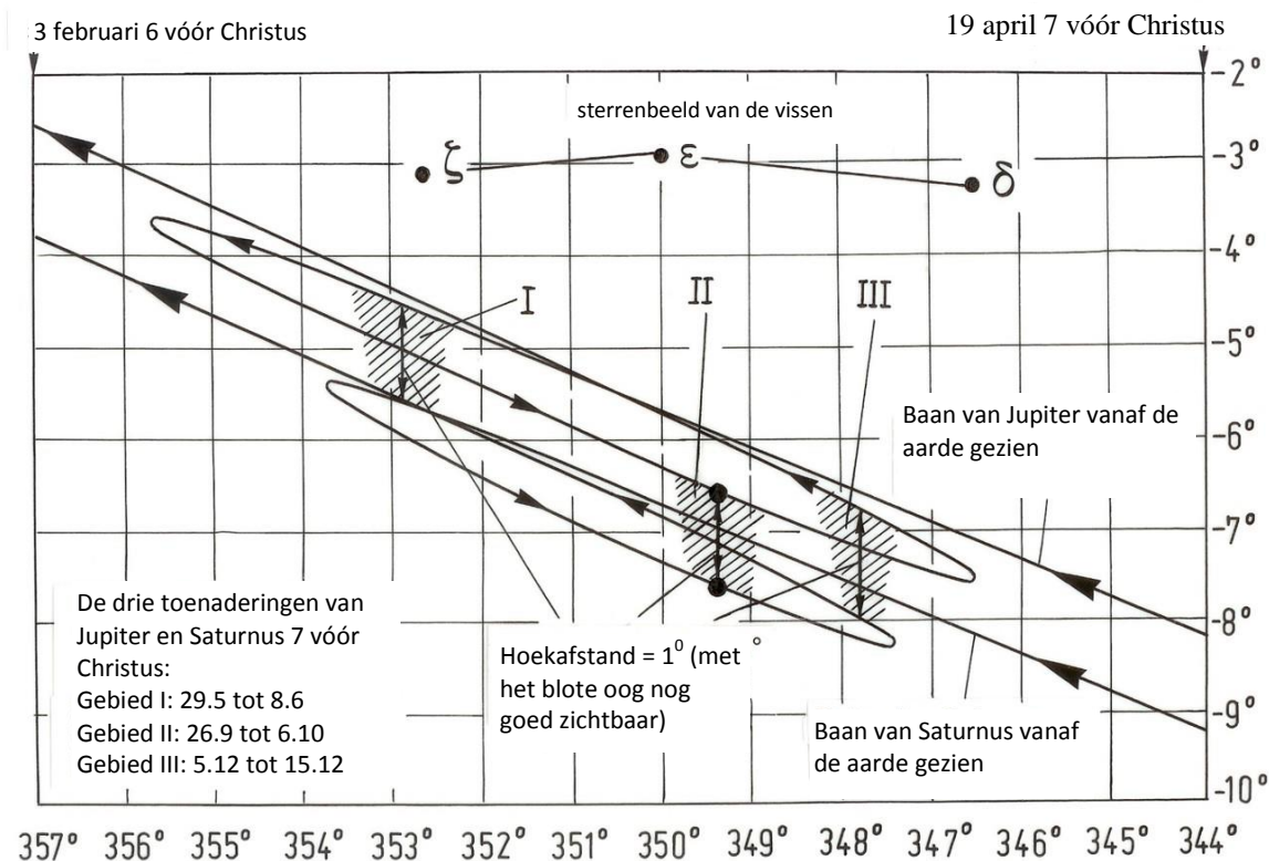
Foto 5: Vanuit de aarde gezien voeren de banen van Jupiter en Saturnus staartbewegingen uit. Bij de drievoudige samenstand van Jupiter en Saturnus in het jaar 7 vóór Christus, bedroeg zelfs in de drie tijden van de toenadering ( I, II en III) de afstand een graad en dat zijn twee diameters van een volle maan.
