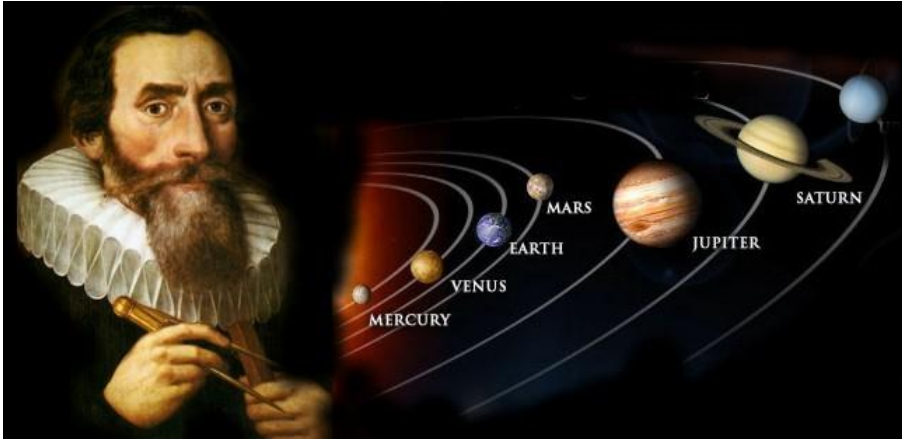
Foto 4: Johannes Kepler (1571-1630), keizerlijke wiskundige en hofastronoom
